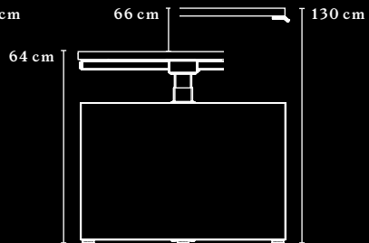
Three-part column, electrically height adjustable Colonne en trois parties, réglable électriquement en hauteur
