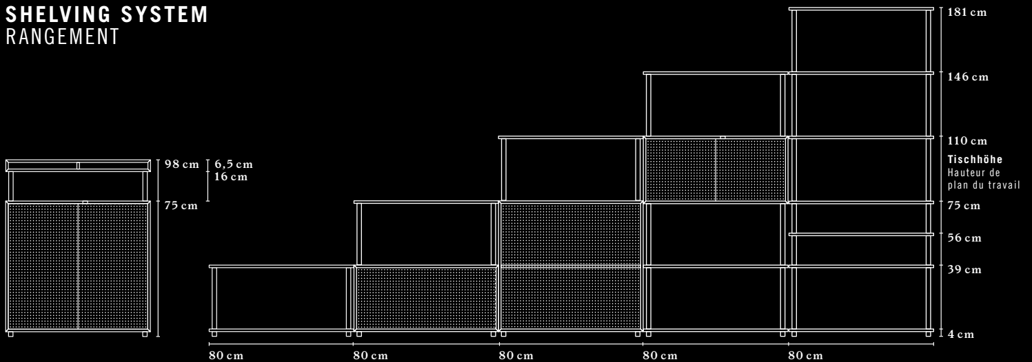
SHELF ETAGERE
