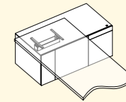
SIDEBOARD FÜR 90°-TISCHANBINDUNG SIDEBOARD FOR 90° DESK CONNECTION B/L: 128 / 145 / 165 / 185 H: 58 / 60 / 62 T/P: 54,5 / 60 / 90
