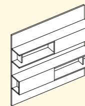
CABINET OFFEN CABINET OPEN B/L: 160-200 H: 38,5 T/P: 38,3
